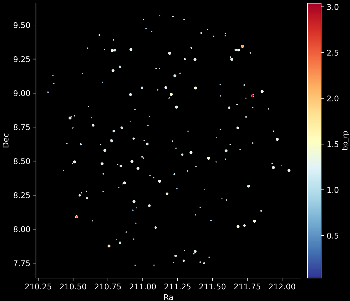
GALAH DR4 Field: [4501] Stars: 163
