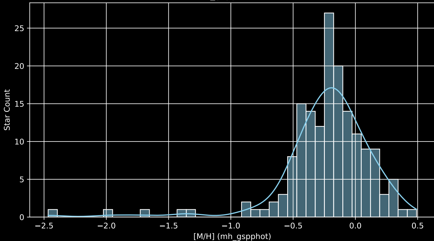
GALAH DR4 Field: [4501] [M/H] (mh_gspphot) (n= 163)
