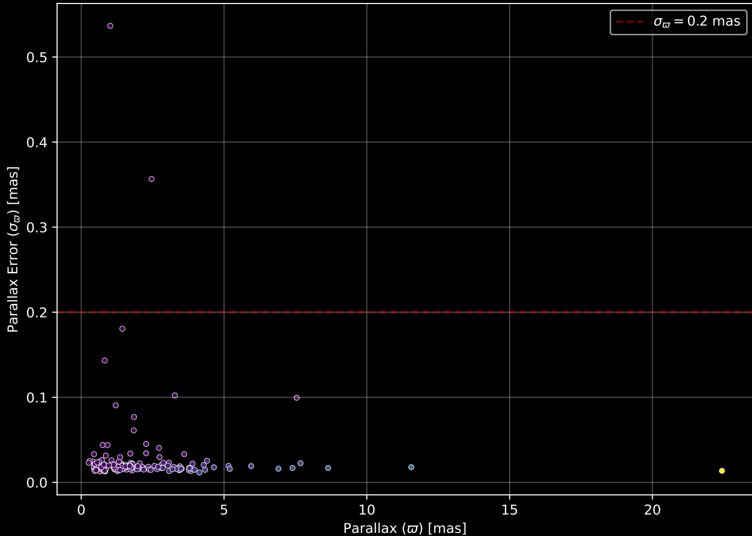
GALAH DR4 Field: [4501] Parallax Quality (n= 163)
