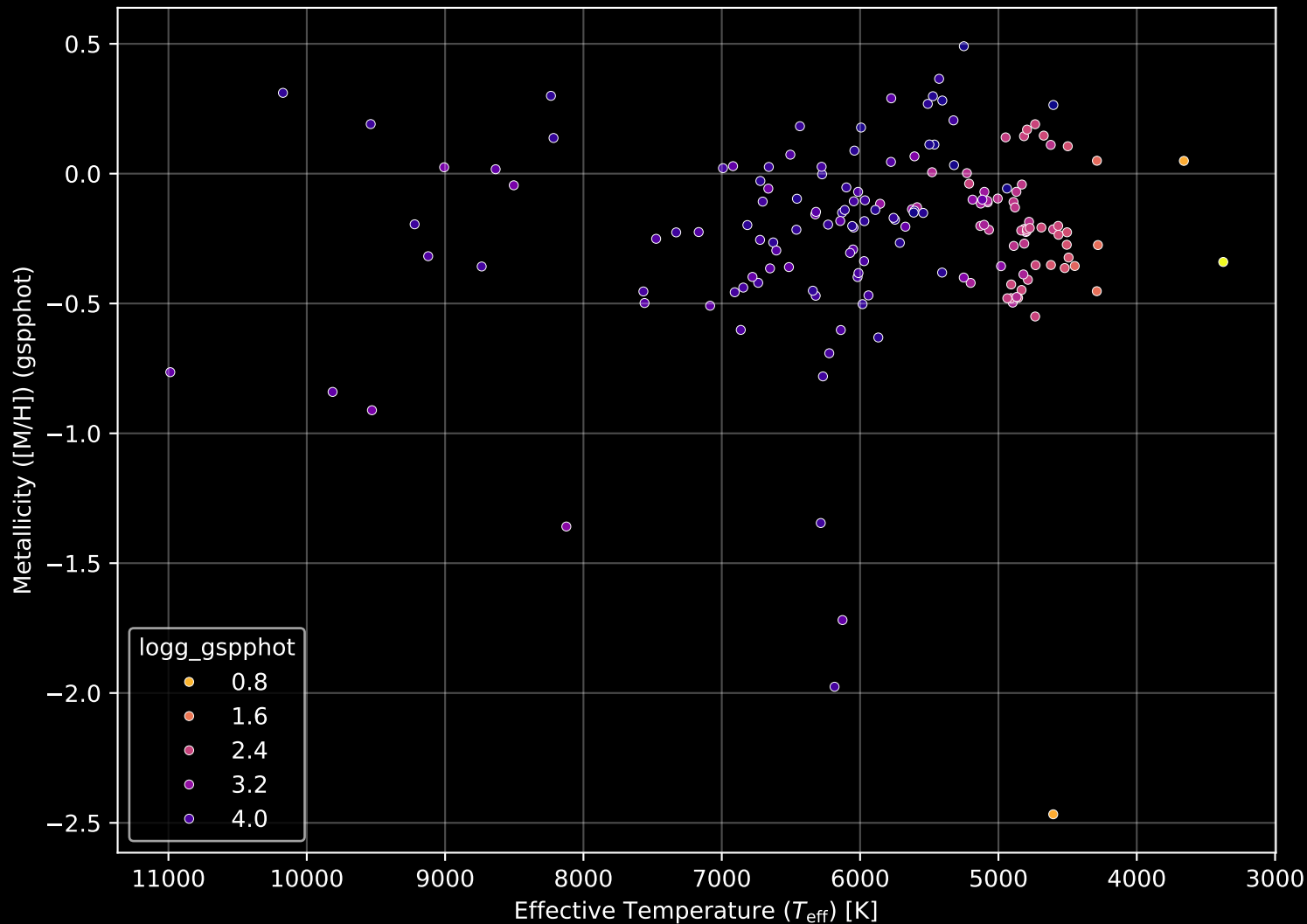
GALAH DR4 Field: [4501] Stellar Population Parameters (n= 163)
